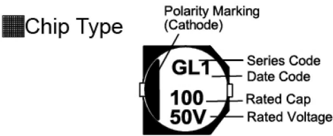
Fig.1 ØD=6~10mm
