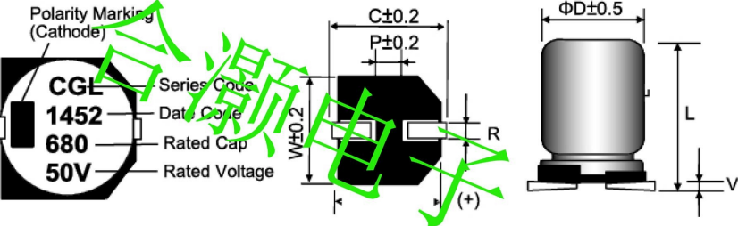
Fig.2 ØD≥12.5mm
